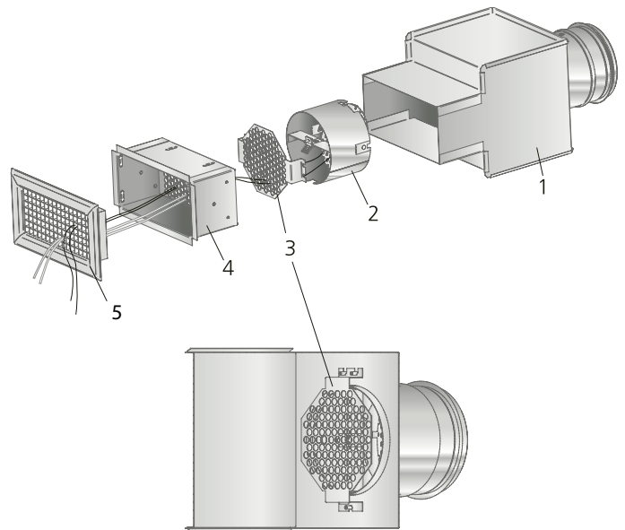
Abbildung 2. Montage, Einregulierung Sicherung von Klappeneinsatz (2) am Kanalananschluss sowie Sicherung des achtkantigen perforierten Blechs (3) am Kanalan- schluss.
