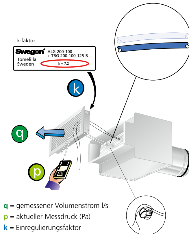
Abbildung 1. Einregulierung Messung mit zwei Schläuchen gemäß C122.
