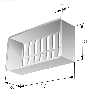
Abbildung 6. Befestigungsrahmen mit Schiebeklappe FHA (1.) Nom. -3 mm.
