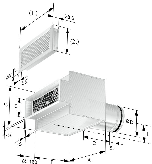
Abbildung 4. ALG (1.) Nominelle Breite + 30 mm
