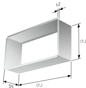
Abbildung 5. Befestigungsrahmen FHB (1.) Nom. -3 mm.
