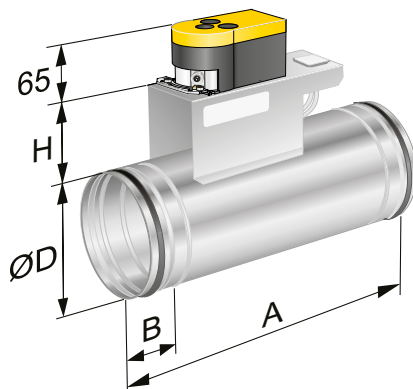
Abbildung 4. Maße (mm), CRM mit Motor.
