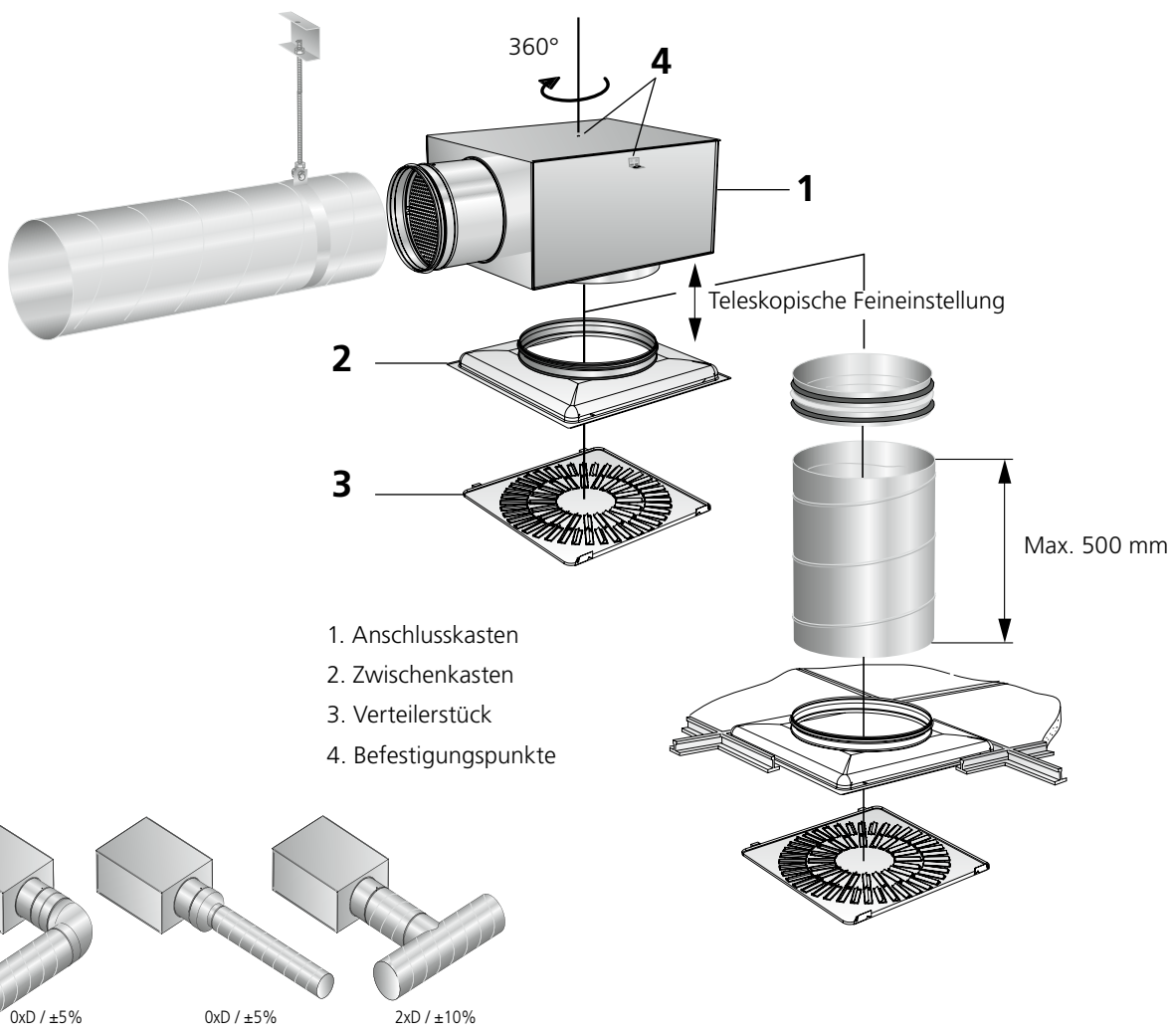
Abb. 2. Montagealternativen.
