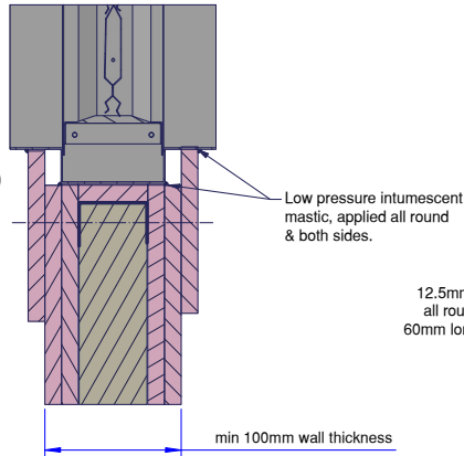
SECTION D-D
