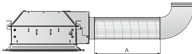
Figur 25. Måttskiss, långsidesanslutning med böj
