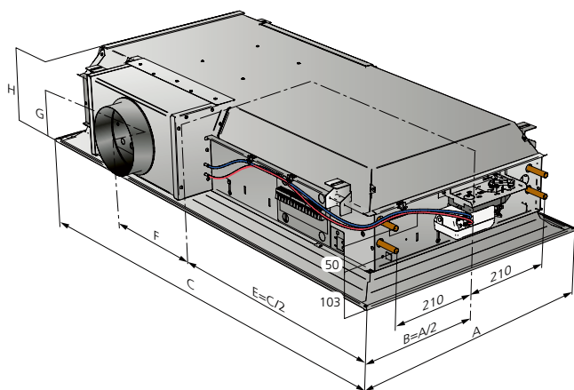
Figur 26. Måttskiss - långsidesanslutning (I exemplet visas längd 1200 med luftanslutning på sidan 4).
