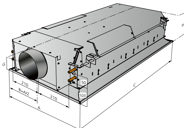
Figur 27. Måttskiss - kortsidesanslutning (I exemplet visas längd 1200 med luftanslutning på sidan 1).
