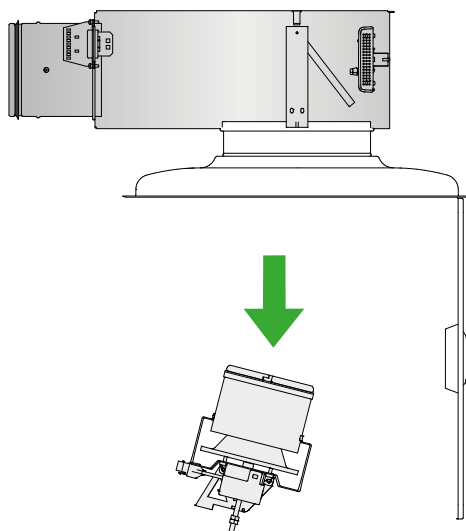
Abb. 10. Demontage des Klappeneinsatzes. Wiedermontage in umgekehrter Reihenfolge.
