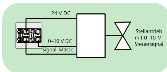
Anschluss eines Stellantriebs mit 0–10-V-Steuersignal. Achtung! 24-V-DC-Versorgung
