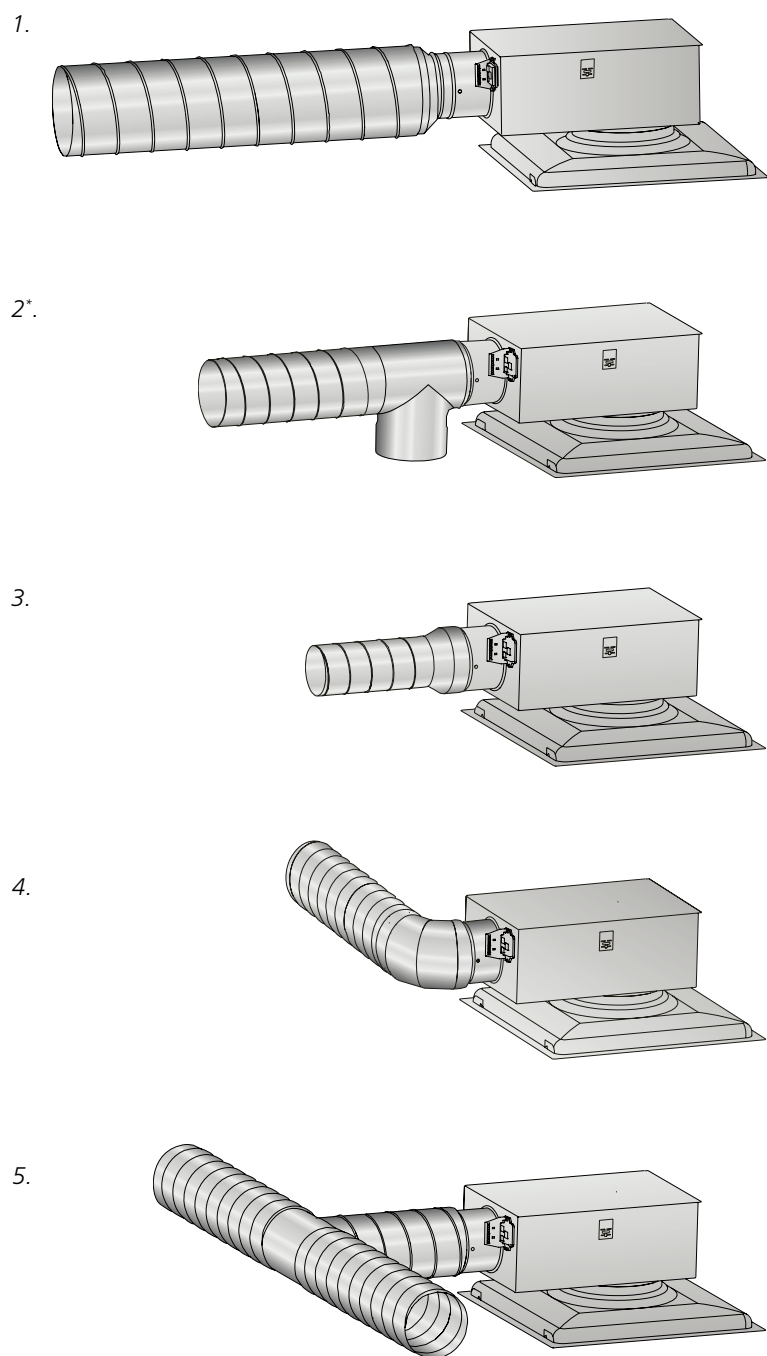
Abb. 5. Anforderung an gerade Strecken.
