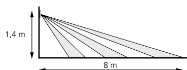
Figur 1. Detekteringsområde, väggmontage.
