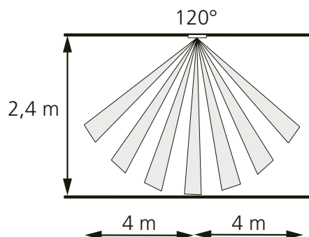
Figur 3. Detekteringsområde, loftmontage.
