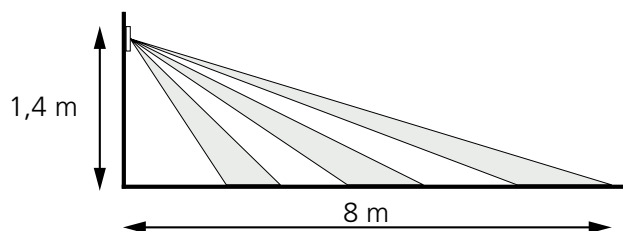
Figur 2. Detekteringsområde, veggmontering.
