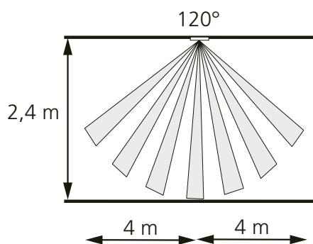
Figur 3. Detekteringsområde, takmontering.
