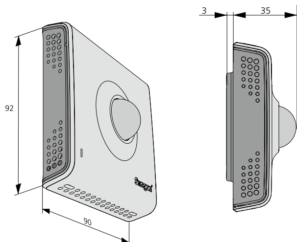
Figur 4. Mått, WISE OCS.
