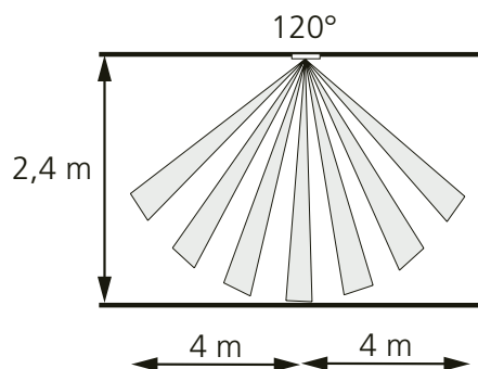
Figur 3. Detekteringsområde, takmontage.
