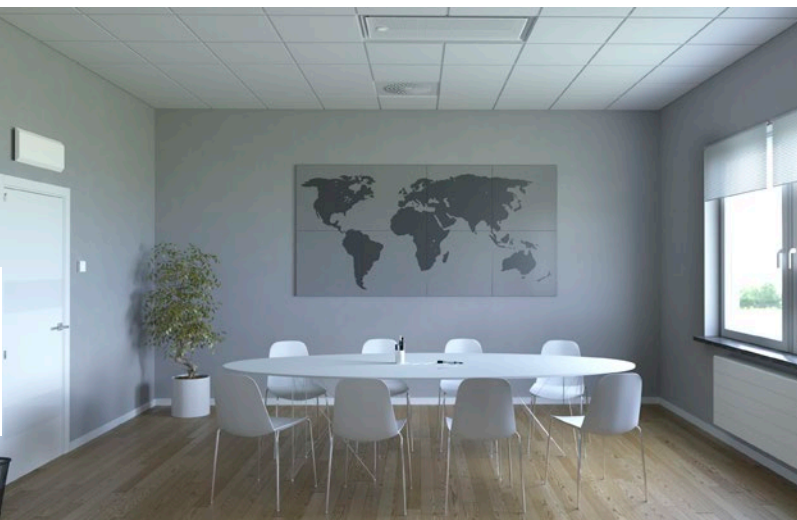
Konferenzraum mit Sollwertumschalter und bedarfsgesteuerter Luftregelung sowie wasserbasierter Kühlung und Heizkörpersteuerung.
