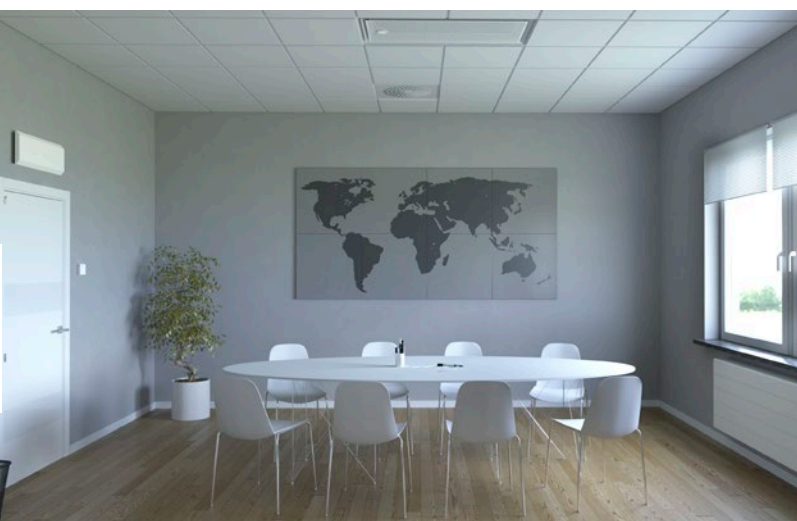
Konferanserom med børverdiratt og behovsstyrt luftregulering samt vannbåren kjøling og styring av radiator.
