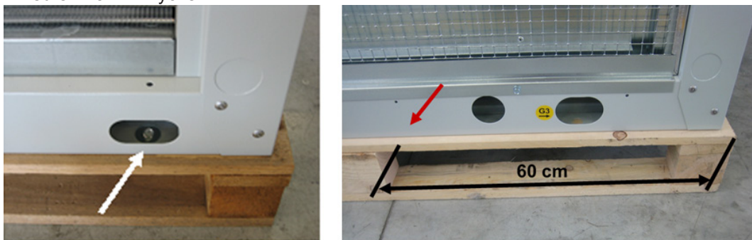
Fig. 7 Detaljer över skruvlägen för fastsättning vid pallens
