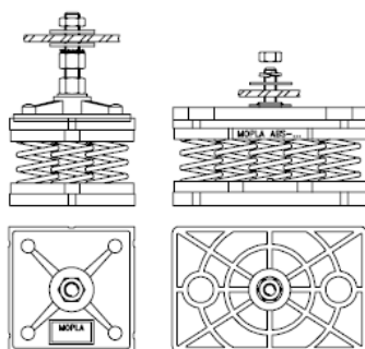
Fig. 11 Vibrationsskydd med fjädring
