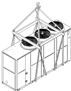
Fig. 6 Lyft med kran
