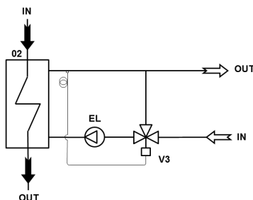
Fig. 1 Installationsschema för 3-vägsventil
