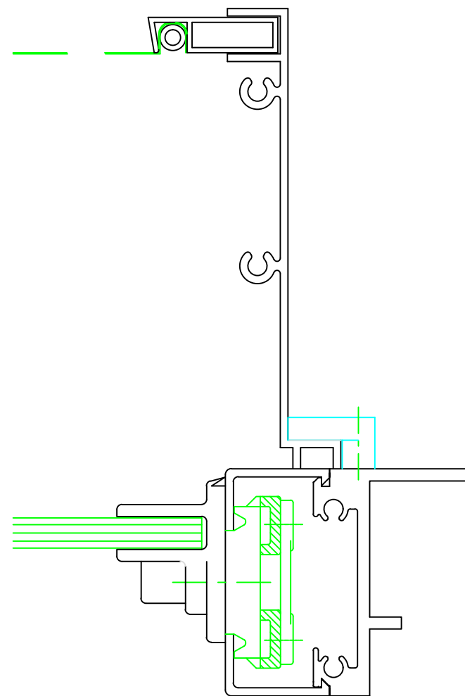
UN-EQUAL JAMB
