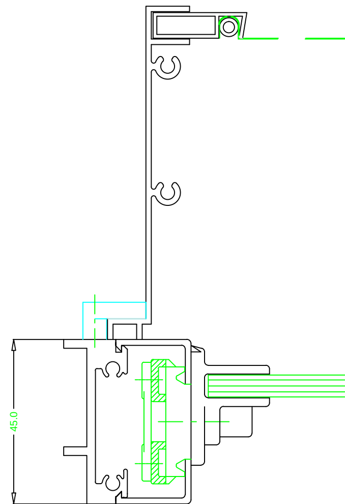
EQUAL JAMB
