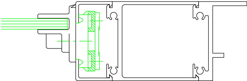
ACTUATOR JAMB
