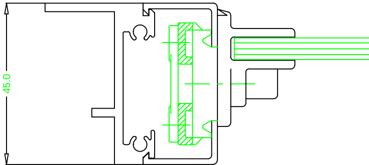
STD JAMB
