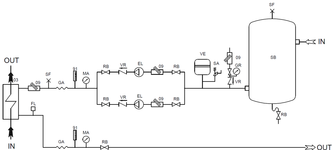
Abb. 12 Empfohlener Wasserkreislauf
