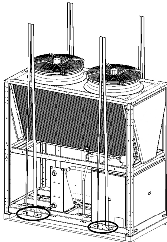
Abb. 7 Detail des Hebens mit Hebeseilen
