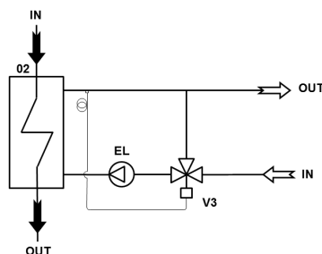
Abb. 1 Installationsschema 3-Wege-Ventil
