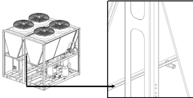
Abb. 3 Position Kondenswasserablass
