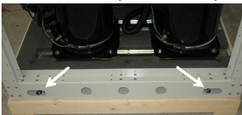
Abb. 6 Besondere Positionen der Schrauben zur Befestigung an der Palette
