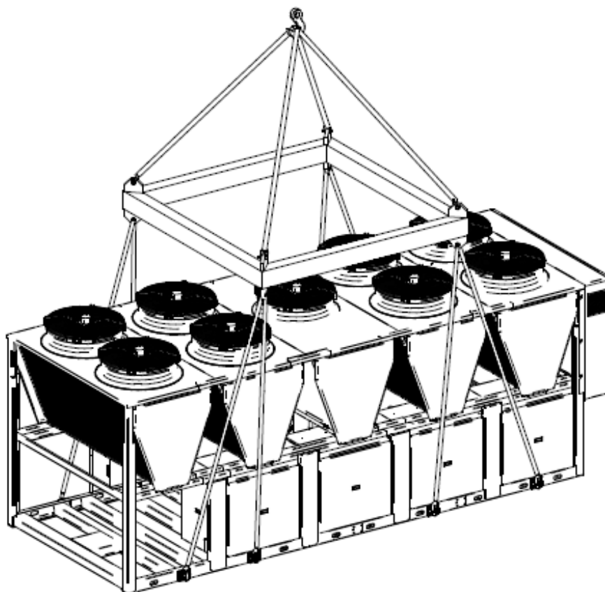
Abb. 5 Heben der Einheit mit Hehebügeln
