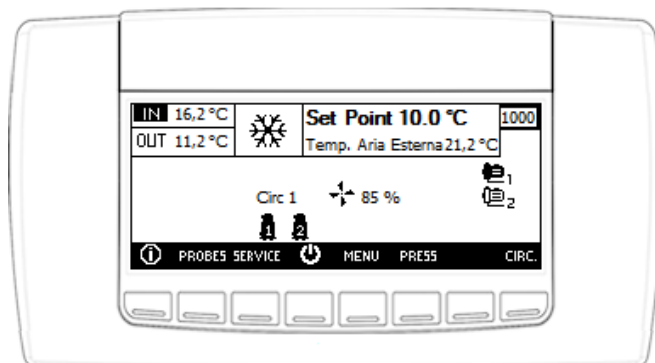
Abb. 9 Display programmierbare Steuerung
