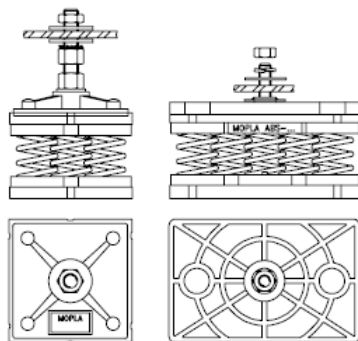
Abb. 11 Schwingungsdämpfer mit Feder
