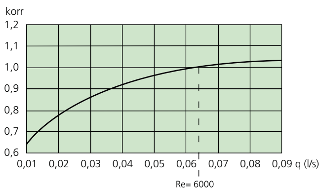
Diagram 1b: Vattenflöde – kapacitetskorrektion, kyla
