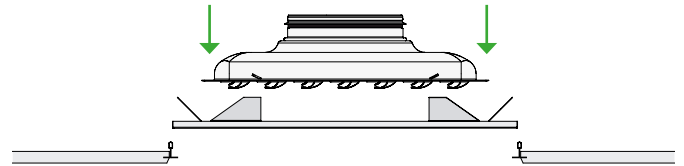
Kuva 1. ADAPTERin ja ilmalaitteen 500 asennus.
