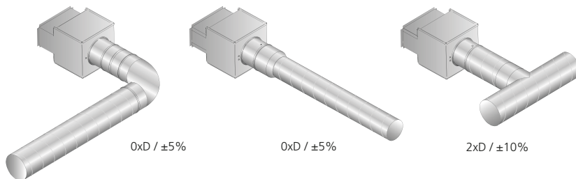
Kuva 3. Asennusvaihtoehdot, koskee kaikkia liitäntöjä (B, K, L)
