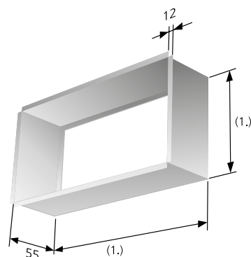
Kuva 5. Kiinnityskehys FHB. (1.) Nim. -3 mm.
