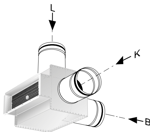
Kuva 7. TRG:n liitännävaihtoehdot B = Liitäntä takaa K = Liitäntä päädystä L = Liitäntä pitkältä sivulta
