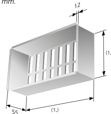
Kuva 6. Kiinnityskehys, jossa säätöpelti FHA. (1.) Nim. -3 mm.
