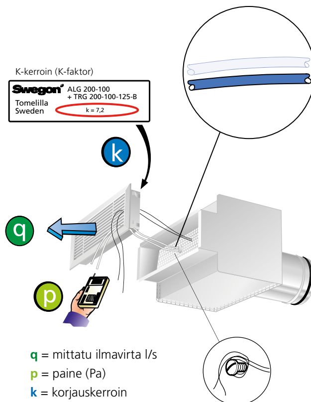
Kuva 1. Sääto. Mittaus kahdella letkulla menetelmän C122 mukaisesti.
