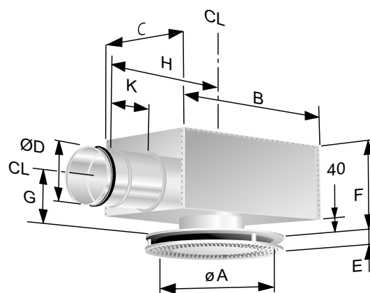
Abbildung 4. CDD/CDR + ALS
