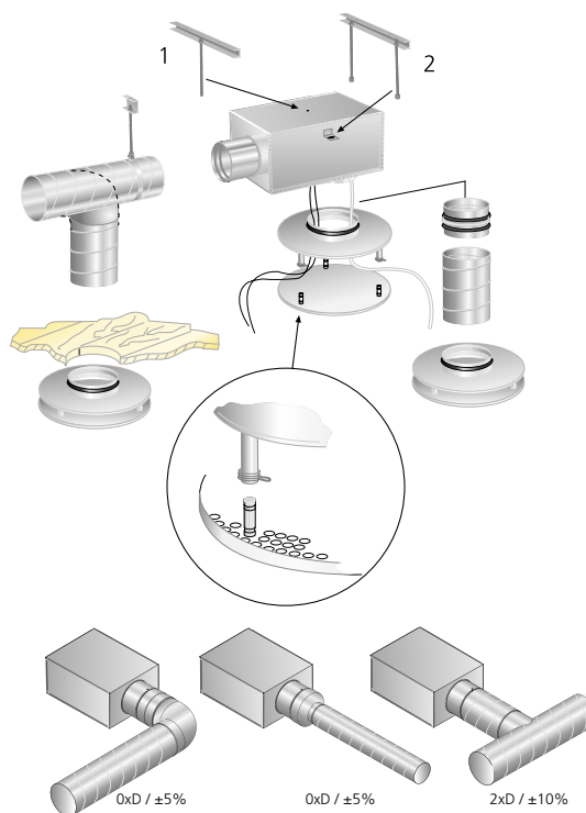
Abbildung 2. Montage
