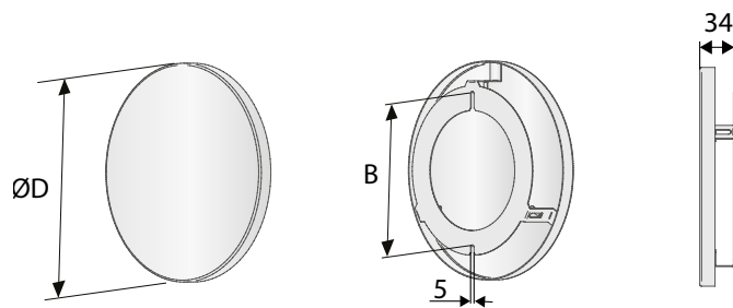
Figur 4. CIRCO, mått.
