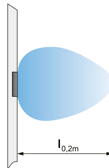
Abb. 7. Isotache. Standard Verteilungsbild, kurze Luftstromlänge.
