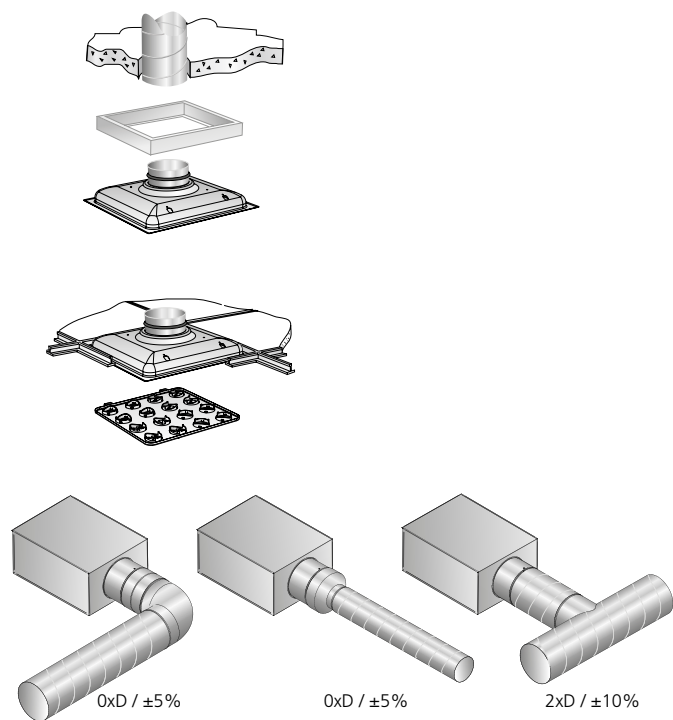
Kuva 3. Asennusvaihtoehto.
