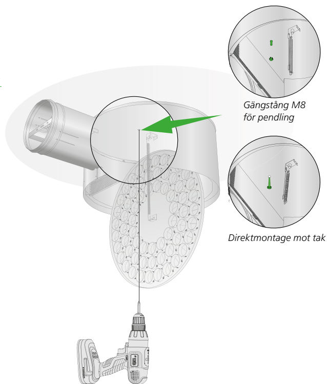
Figur 1b. Alternativ montering i förstansat Ø10 mm hål.
