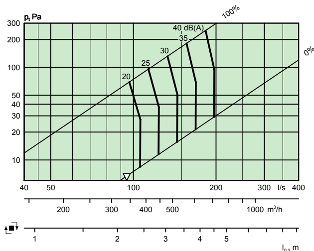
EAGLE S 315 + ALS 250-315
