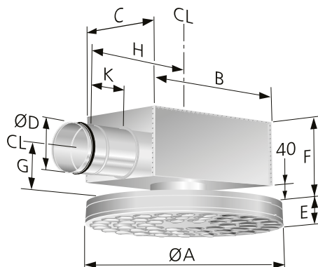
Figur 3. EAGLE S med ALS.
