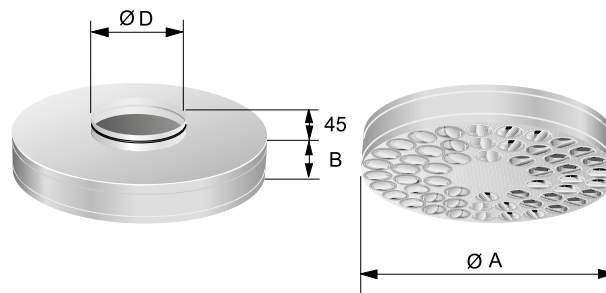
Figur 2. Dyseventil EAGLE S.
