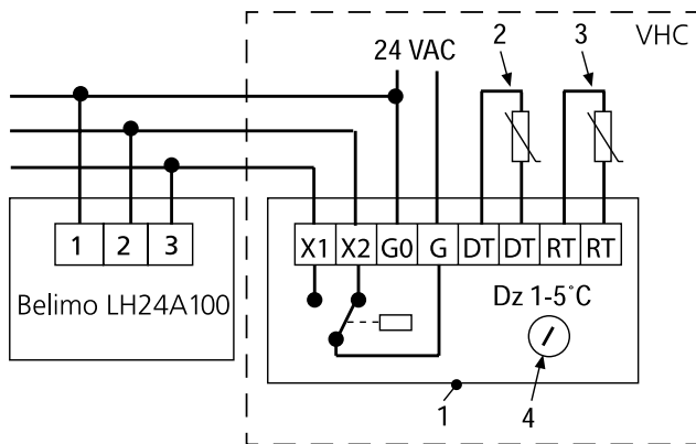
Figur 5. Kopplingsschema visar inkoppling med Belimos spjällmotor mot VHC. OBS! Finns endast med 24 V AC spänningsmatning.
