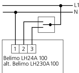
Figur 4. Kopplingsschema för FALCON C med motor - Motorstyrning med 3-punktsreglering. Omkopplare ingår ej.
