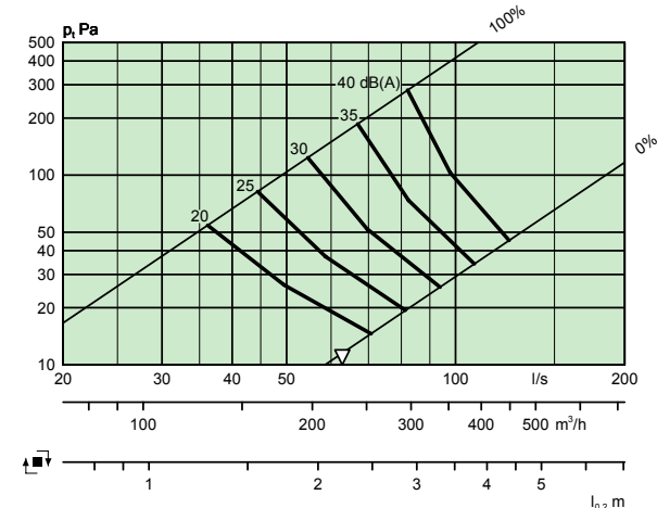
LOCKZONE C 250-600 + ALS 160-250 – To trin
