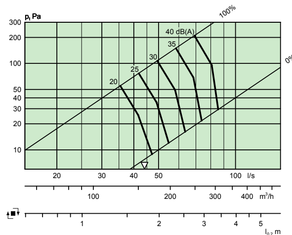
LOCKZONE C 200-600 + ALS 160-200 – Et trin
