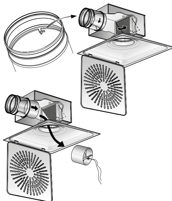
Figur 4. Afmontering af spjæld.
