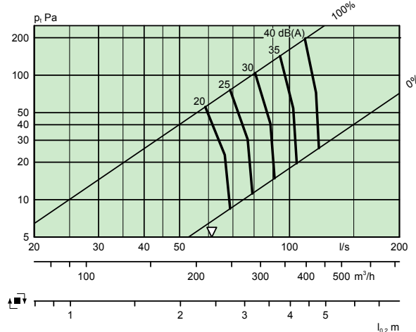
LOCKZONE C 250-500+ALS 200-250 – Et trin
