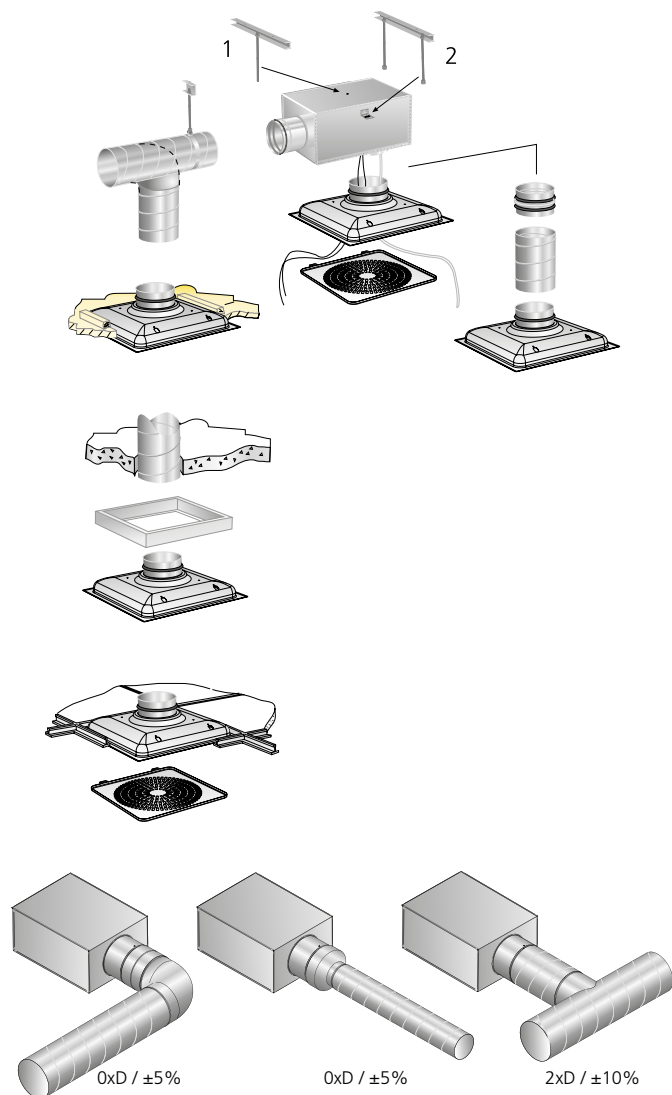
Figur 2. Monteringsalternativ.
