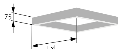
Figur 8. Skørt SAR K.
