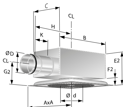
Figur 7. LOCKZONE Ceiling med ALS. Lav konstruktionshøjde.
