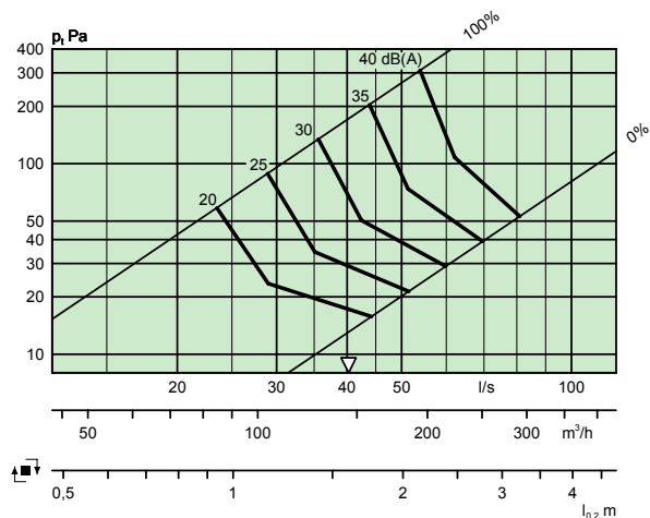
LOCKZONE C 200-500 + ALS 125-200 – To trin
