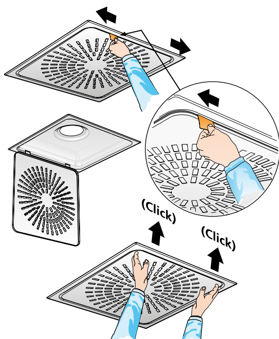
Figur 1. Quick Access, afmontering af armaturfront.
