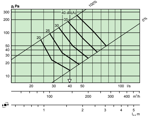
LOCKZONE C 200-600 + ALS 125-200 – To trin
