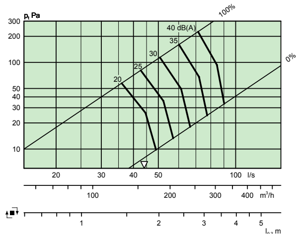
LOCKZONE C 200-500 + ALS 160-200 – Et trin
