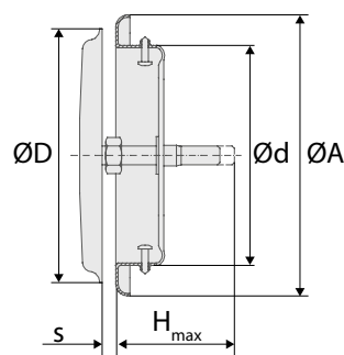
Figur 6. TRAC, mått.
