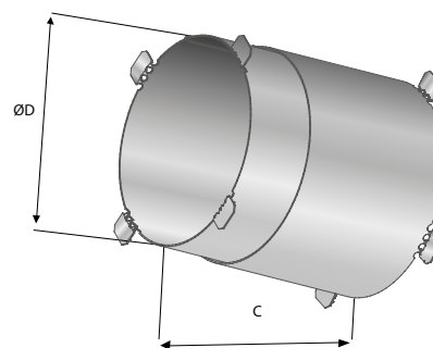
Figur 5. VGC, mått.
