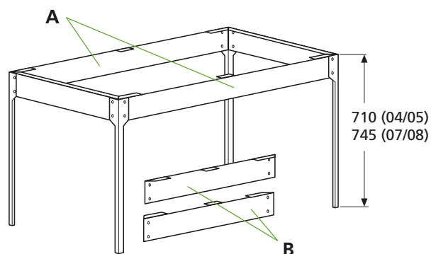
Piedistallo per unità GOLD RX/SD delle misure 004/005 e 007/008.
