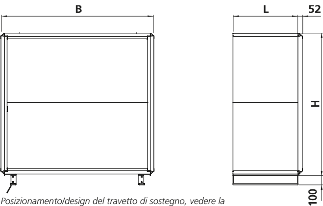
Posizionamento/design del travetto di sostegno, vedere la taglia equivalente dell'unità di trattamento aria GOLD.
