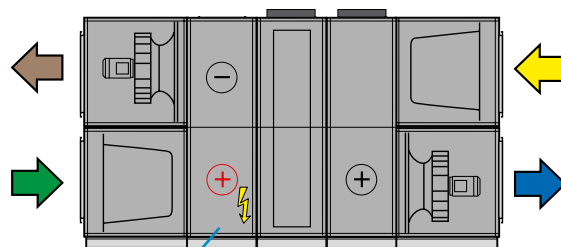
Elektrisk luftvärmare placerad i RX/HC (tillbehör)
