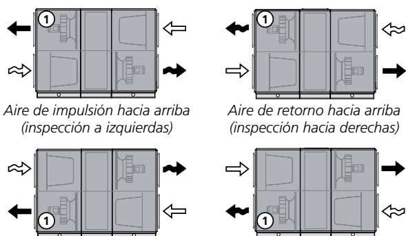
Aire de impulsión hacia abajo (inspección a izquierdas). No hay RX tamaños 004-008 en caja común.
