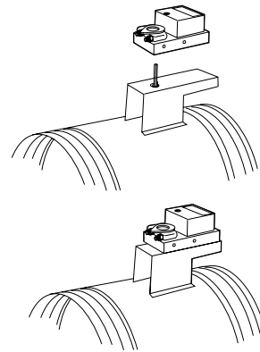
Abbildung 3. Motor montage, größe 100-400.
