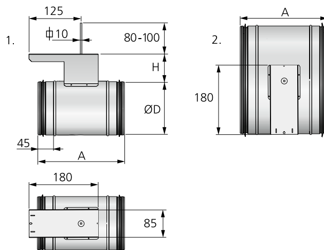
Abbildung 11. Maße (mm), CRT.
