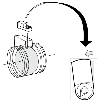
Abbildung 4. Motor montage, CRT, größe 500 und 630. Zuerst schliessen Sie die Klappe vollständig, dann montieren Sie den Stellmotor spannungsfrei auf der Klappenwelle und befestigen diesen. Jetzt öffnen Sie die Klappe um 5° am Stellmotor und verriegeln diesen wieder.
