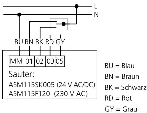
Abbildung 6. Schaltplan Sauter, 3-punktregelung.
