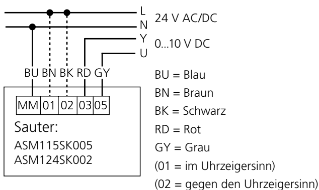
Abbildung 7. Schaltplan Sauter, 0-10 V stufenlos / modulierende Regelung.
