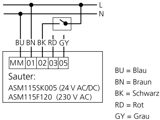
Abbildung 5. Schaltplan Sauter, 2-punktregelung.
