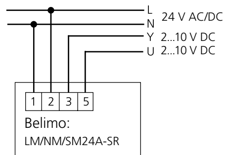
Abbildung 10. Schaltplan Belimo, 2-10 V stufenlos / modulierende Regelung.
