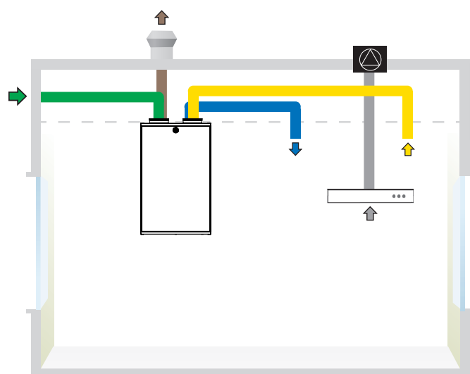
CASA W5 L, kanalanslutningar och spiskåpa anslutna till extern takfläkt.
