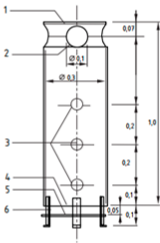
Fig. 2: Simulateur de charge frigorifique (exemple), source: EN 14240:2004 (D)
